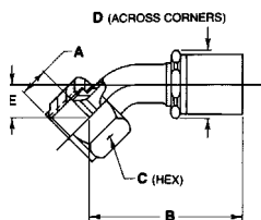
45° ELBOW
