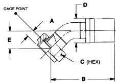
45° ELBOW
